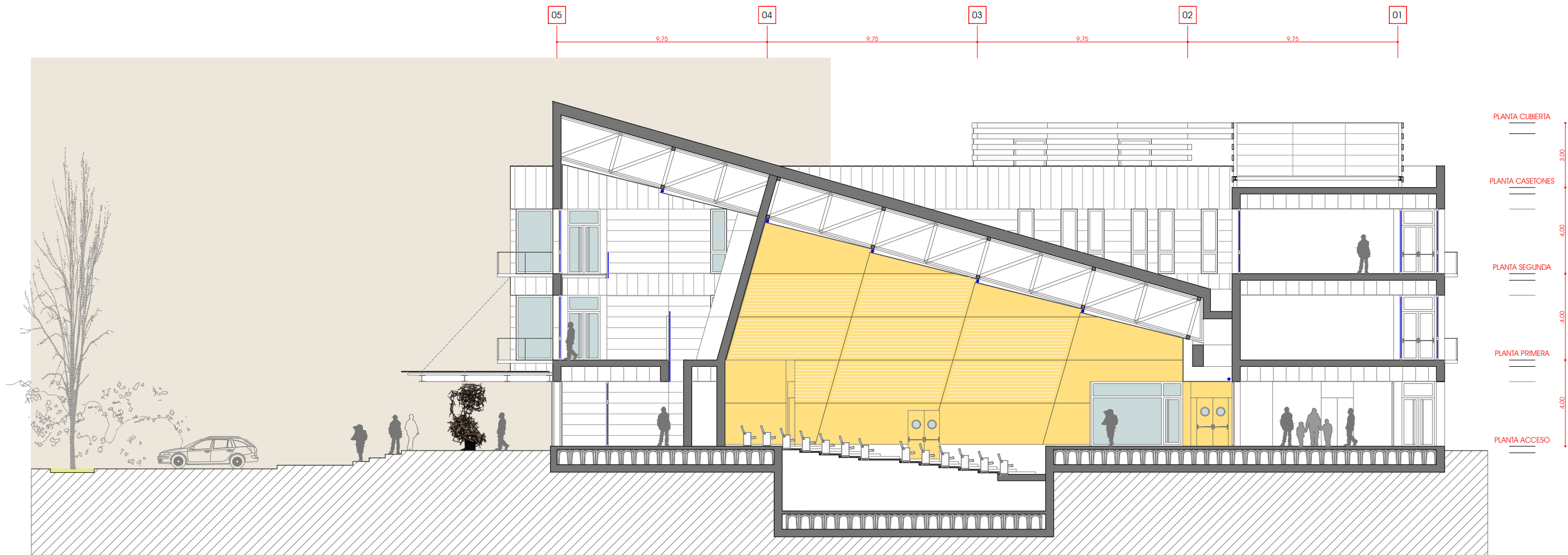
SECCION POR AUDITORIO
